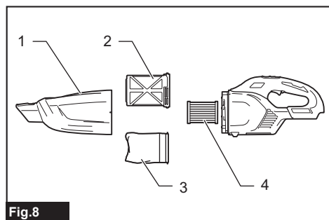
► 1. Bac à poussière 2. Préfiltre 3. Filtre haute performance 4. Filtre HEPA
