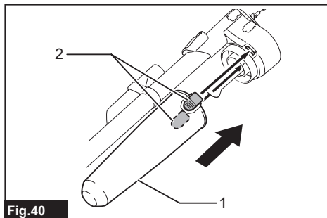
Fig.40 ► 1. Compartiment à poussière 2. Bouton (deux emplacements)
