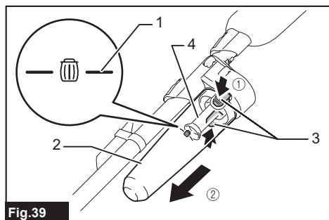
Fig.39 ► 1. Ligne Plein 2. Compartiment à poussière 3. Bouton (deux emplacements) 4. Filtre à tamis
